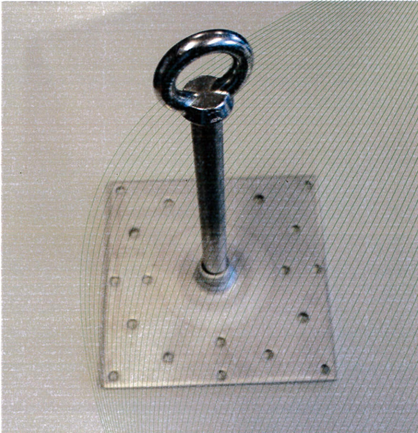
Bild 1: Beispiel der Anschlageinrichtung, Typ: Primo 7 HS
