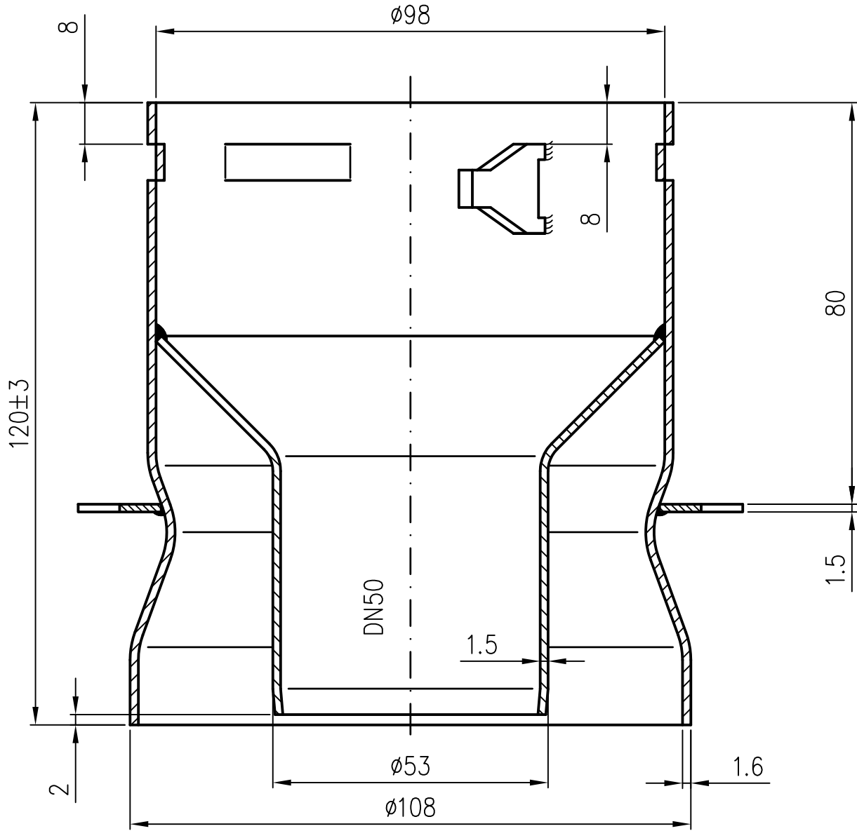
Rohrende DN50 leicht eingezogen
